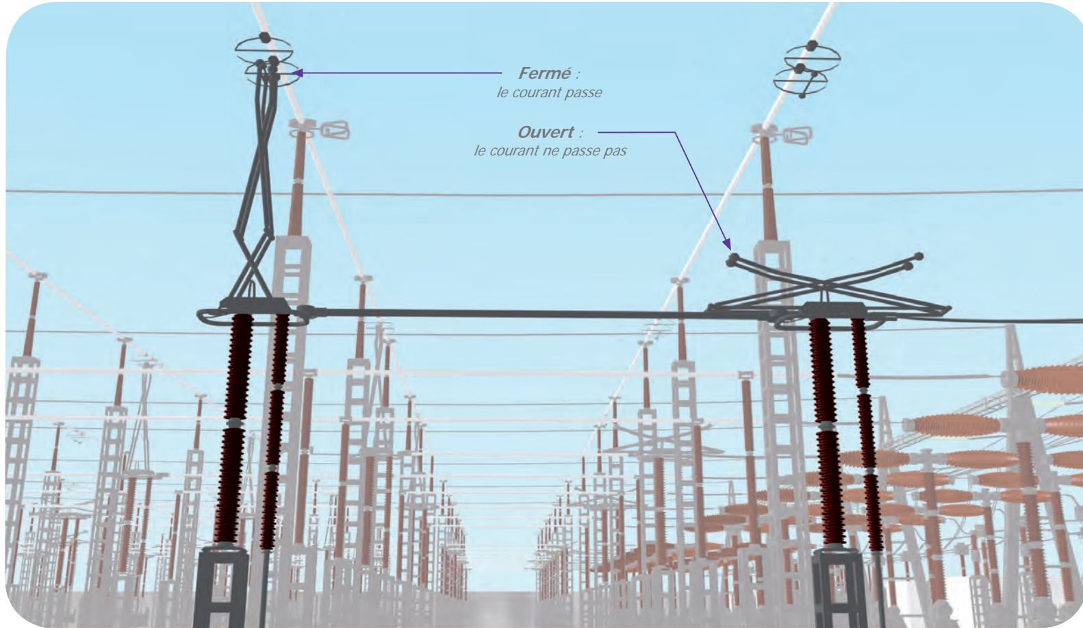
Sectionneur d'aiguillage
